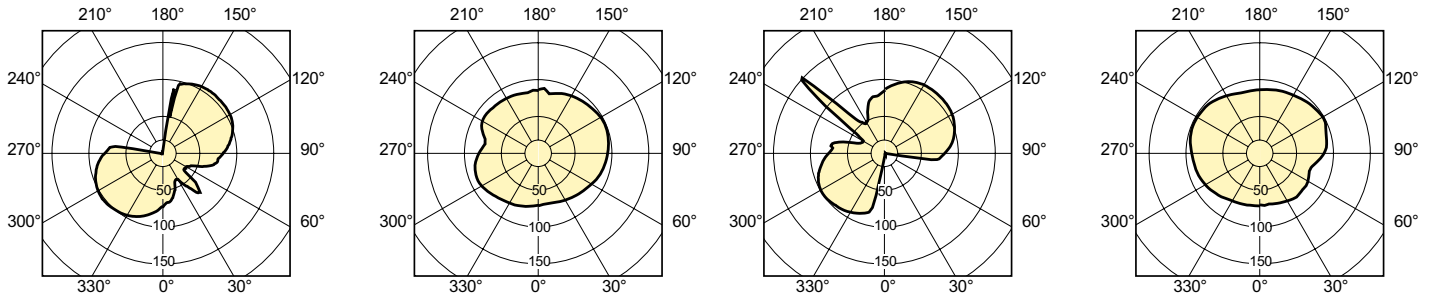
CDM-T 35W /842 lamp 45
