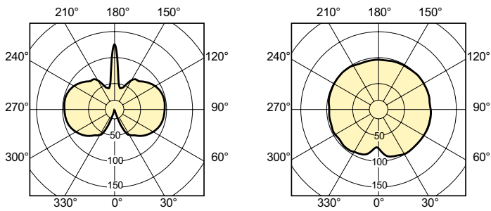
CDM-T 35W /842 lamp down
